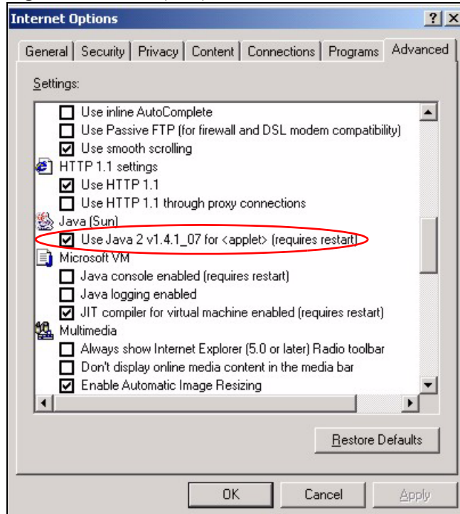
Figure 114 Java (Sun)
